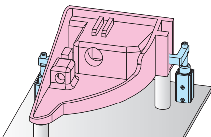
組立ジグ ヘッドランプなど
