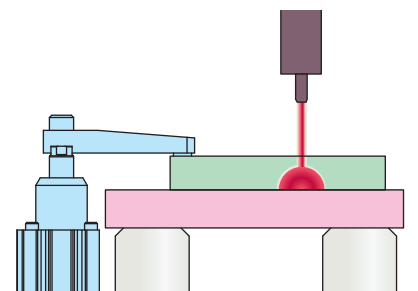
レーザー溶着ジグ 異材接合など
