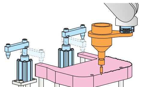
バリ取りジグ 車載成形品など
