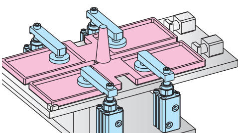
ゲートカットジグ 小型プラスチック製品など
