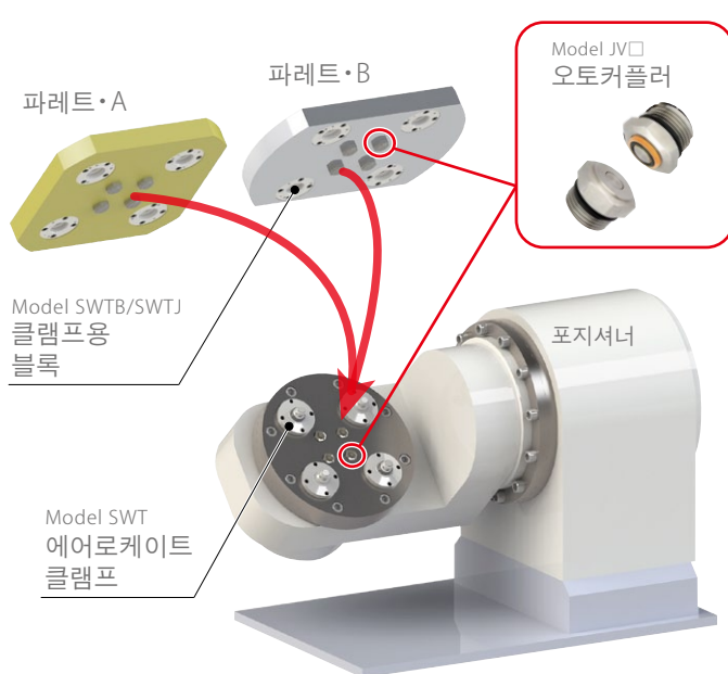
지그 파레트 준비교체
