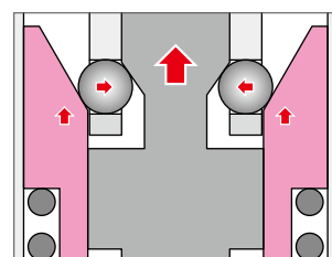
셀프 로크 상태
