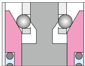
로크 동작 중 (이동스트로크 완료)
