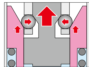
로크 상태 (배력 스트로크)
