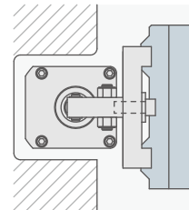
하이파워 에어 클램프
