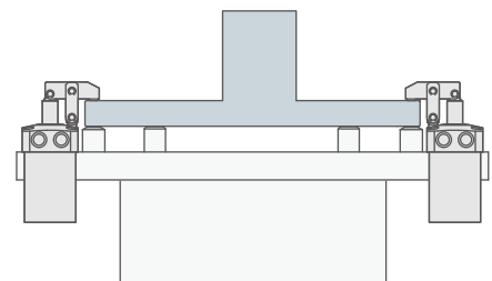
하이파워 에어 클램프
