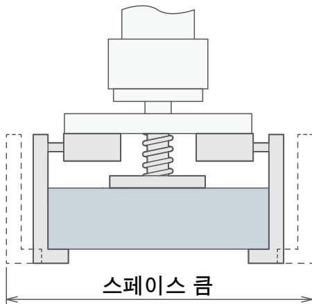
외주를 잡는 직동 실린더
