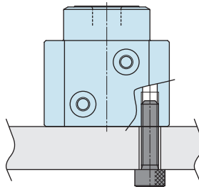
【그림 2 : 밀면 나사를 사용해서 취부】
