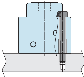
【그림 1 : 상면에서 취부】
