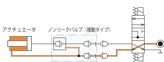
回路例
