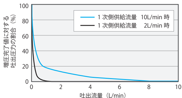
AU2851-0/AU2550-0M□ 2次側吐出流量特性図
