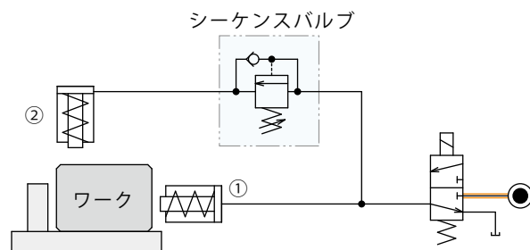
回路例
