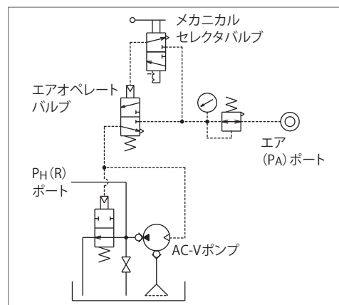
CV5C□0-□-HHR : 回路記号
