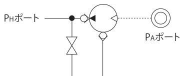
4 回路記号 無記号：標準タイプ
