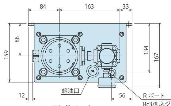
BH ノンリークバルブユニット CCポンプユニット
