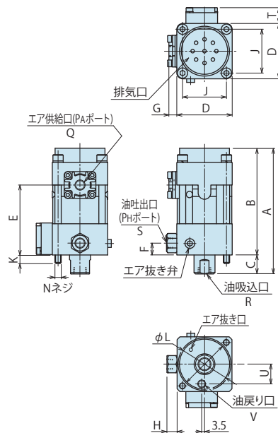
AB-V (バルブ内蔵タイプ)
