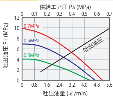
AB7000 計算式 P_H = 59(P_A - 0.04)
