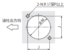
取付穴加工図(共通)
