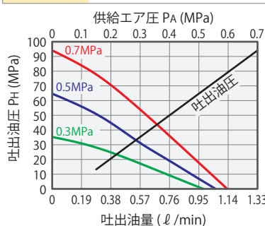
AC9001 計算式 P_H = 147(P_A - 0.06)
