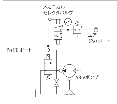
CV2B□0-□-HHR : 回路記号
