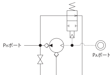
4 回路記号 V：バルブ内蔵タイプ
