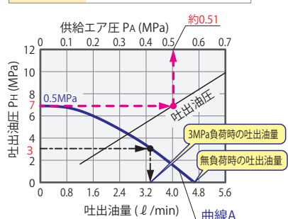
AB4000 計算式 P_H = 15(P_A - 0.04)
