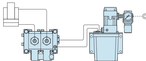
BH ノンリークバルブユニット CBポンプユニット
