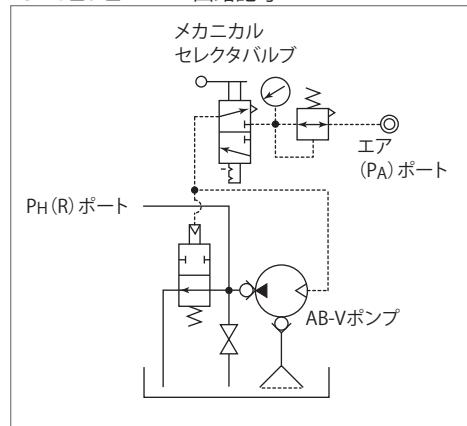
CV2B□0-□-HHR : 回路記号
