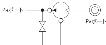
4 回路記号 無記号：標準タイプ
