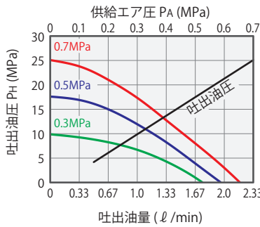
AB6000 計算式 P_H = 38(P_A - 0.04)
