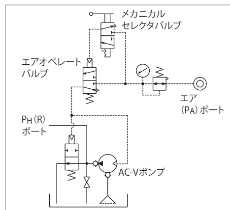
CV5C□0-□-HHR : 回路記号
