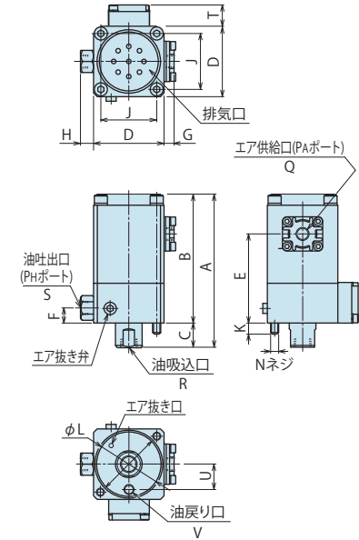
AC-V (バルブ内蔵タイプ)
