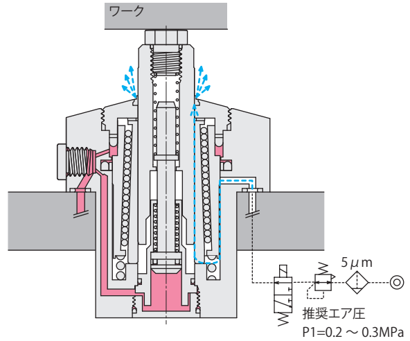
TC プランジャ上昇動作およびロック時 (エア供給入) ※1
