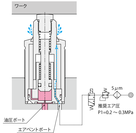
TNE プランジャ上昇動作およびロック時 (エア供給入)※1
