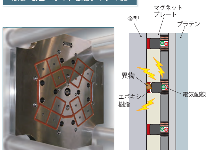
従来品 表面エポキシ樹脂タイプの場合
