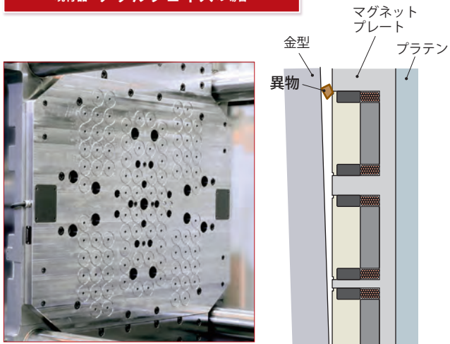
現行品 メタルフェイスの場合
