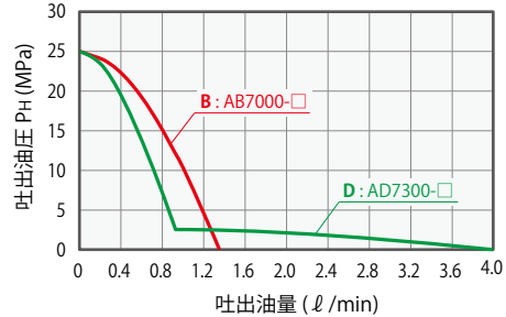
ポンプ性能曲線
