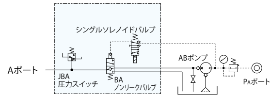
H ダイリフタ用シングルソレノイドバルブ仕様
