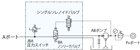
G クランプ用シングルソレノイドバルブ仕様
