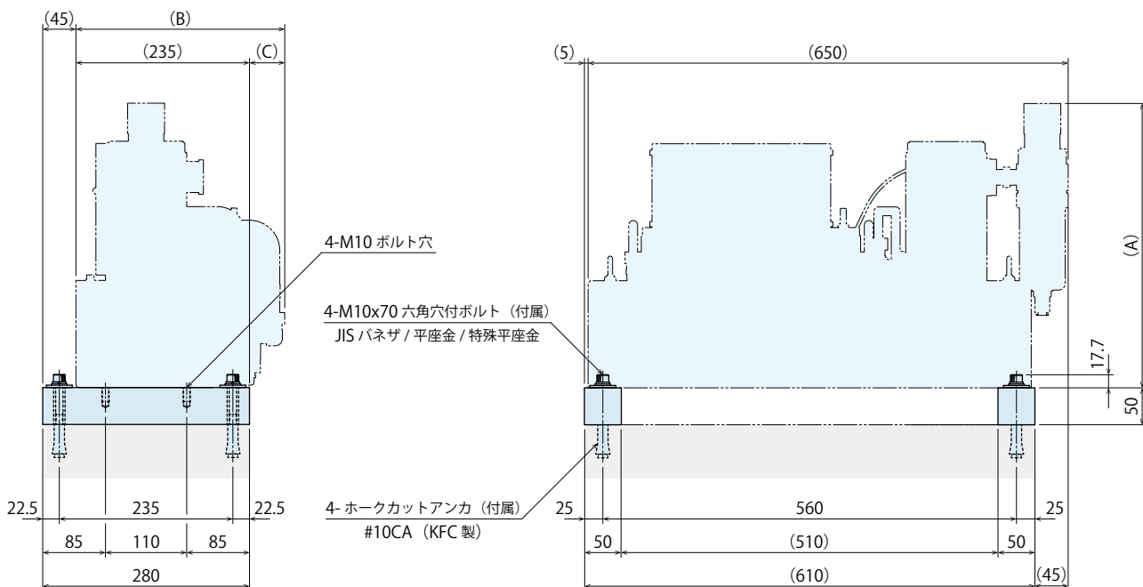
ホークカットアンカ施工寸法
