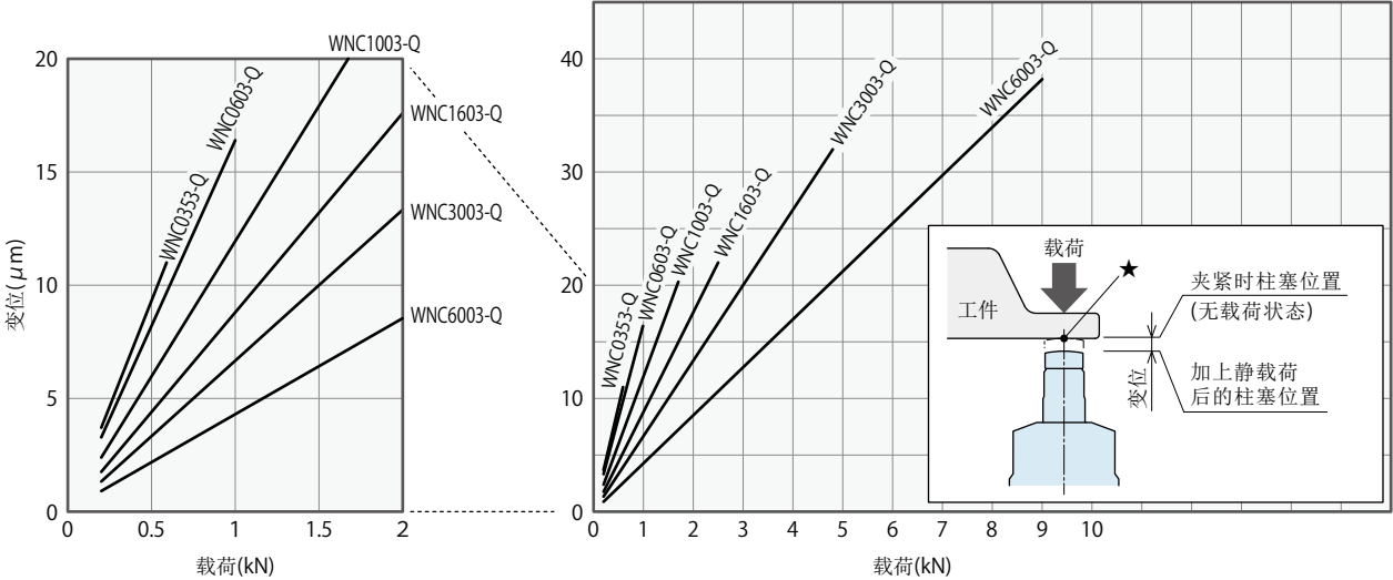
载荷/变位曲线图 ※ 本载荷/变位曲线图表示供给气压为0.7MPa条件下的静载荷下的变位情况。 ★标记部位的凹凸以及因周边夹紧器等引起的工件侧变位不包含在内。
