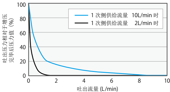
AU2531-0□/AU2530-0M□ 2次侧吐出流量特性图
