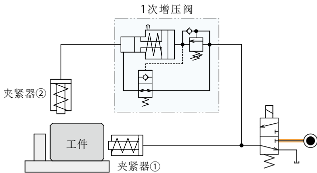
回路实例
