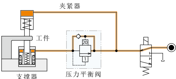
回路实例
