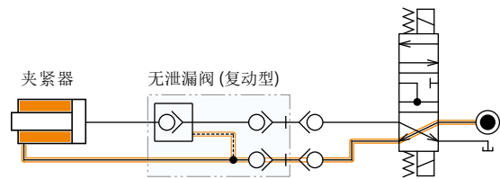
回路范例
