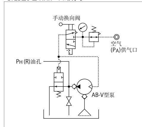
CV2B□0-□-HHR : 回路符号
