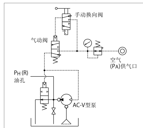
CV5C□0-□-HHR : 回路符号
