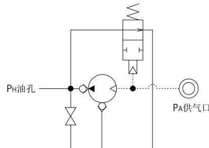
4 回路符号 V: 阀内置型
