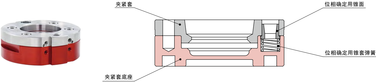
工具适配器 (SMR -T)
