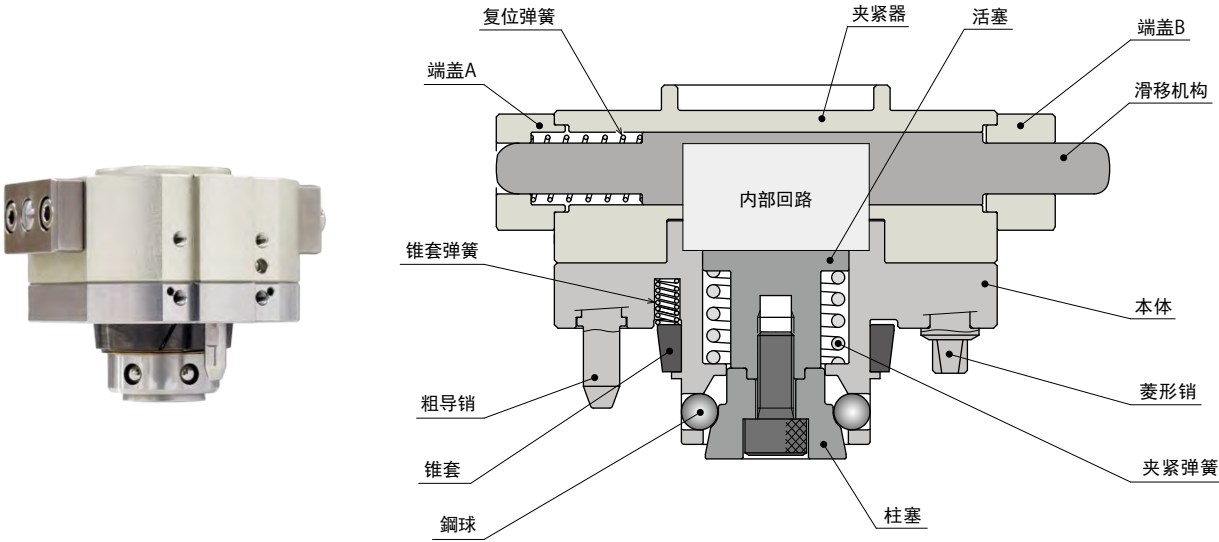
主夹紧器 (SMR -M)
