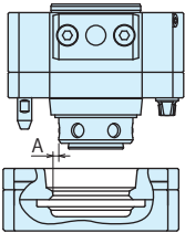
① 水平位置误差
