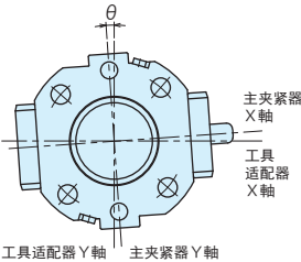
③ 旋转位置误差
