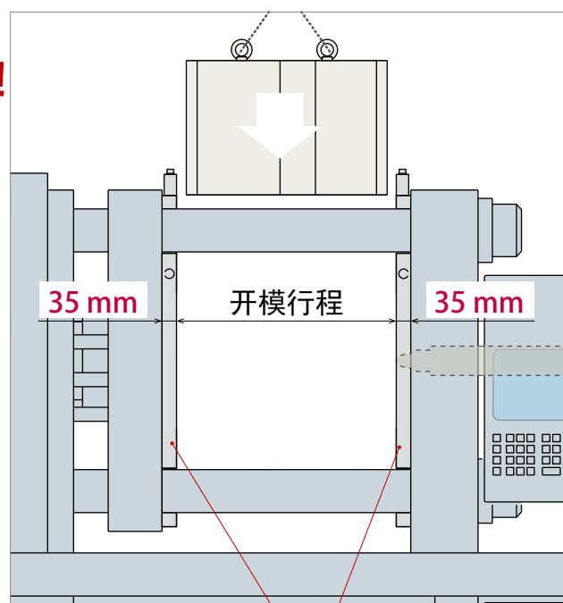
薄型电磁锁模板
