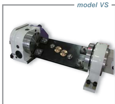
位置決めクランプ+NC円テーブルの パレット交換ジグ
