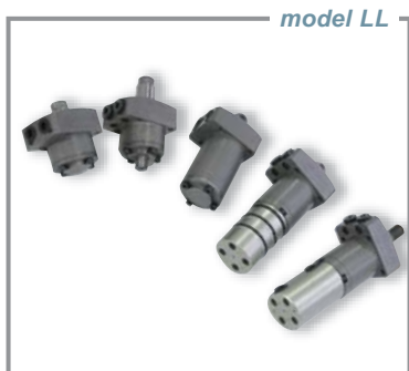
油圧ポート集約タイプ リニアシリンダ
